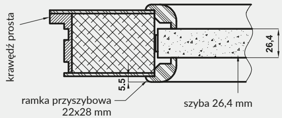
konstrukcja skrzydeł przeciwpożarowych Olimp EI60
