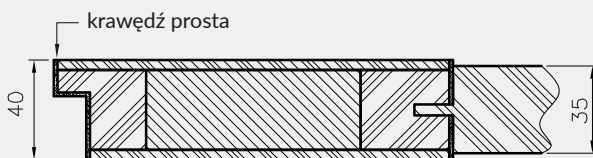
Przekrój poziomy drzwi Tizano
