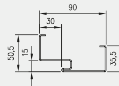
Profil ościeżnicy metalowej
