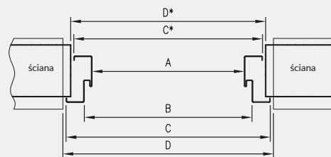
Przekrój poziomy
