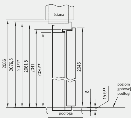
Przekrój pionowy
