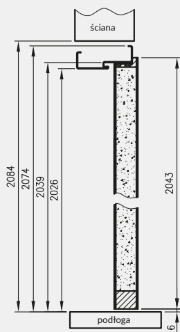
Przekrój pionowy drzwi p.poż.
