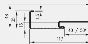
Przekrój ościeżnicy metalowej p.poż. do skrzydeł OLIMP
