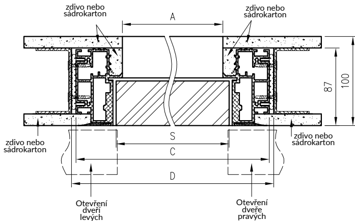
Průřez dveří 50 mm bezfalcové dveře - otevírání ven
