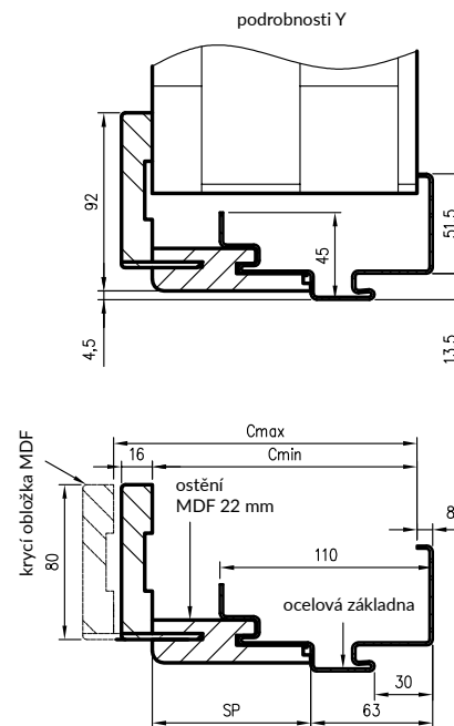
varianty zárubně v závislosti na tloušťce stěny
