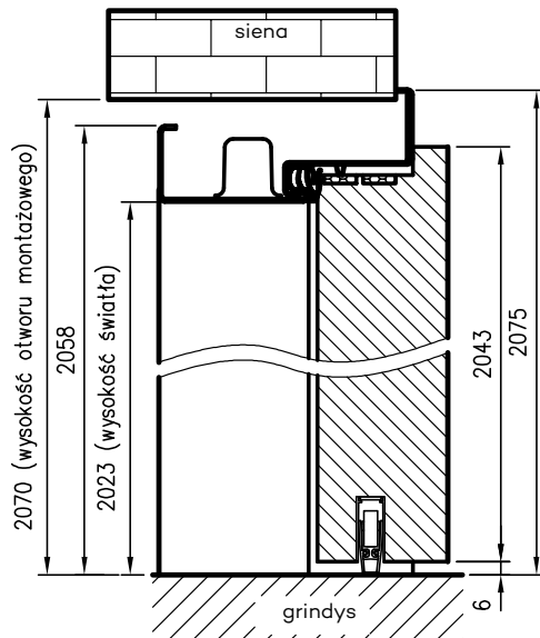
„Olimp EI60“ vienvėrių durų matmenys
