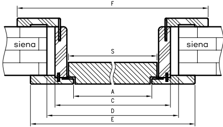
Horizontalus pjūvis ORO
