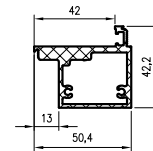
DRE profilis į išorę atsidarančioms lygiabriaunėms durims
