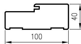
OPB profilis
