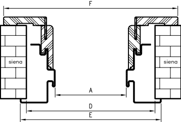
Staktos profilis
