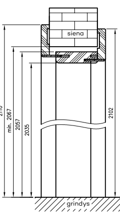
Reguliuojamo tunelio su kamp. T63 vertikalus pjūvis
