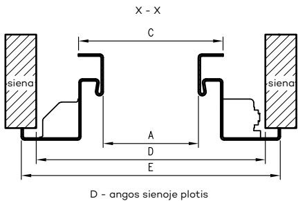
matmenys vienvėrėms durims
