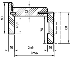
Staktos profilis
