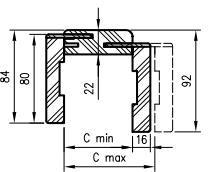
TUN su kamp. T63 pjūvis
