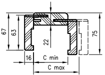
TUN su kamp. T63 pjūvis
