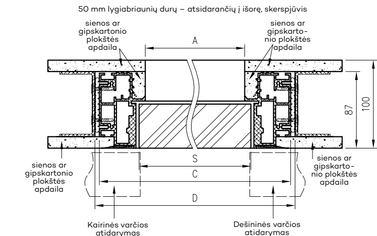
„Profi“ durų pločio matmenys
