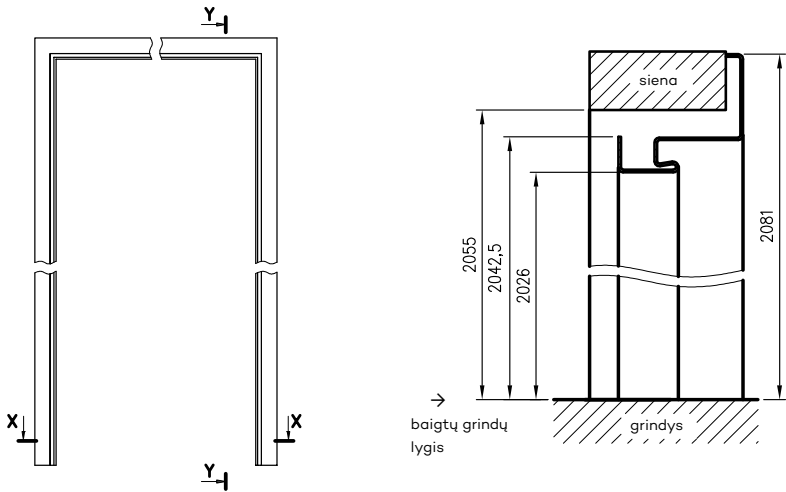
matmenys vienvėrėms durims
