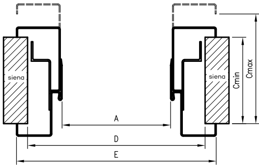
Horizontalus pjūvis OSRB
