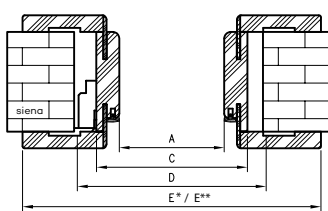
Horizontalus pjūvis OR
