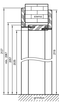
Reguliuojamo tunelio su kamp. T80 vertikalus pjūvis
