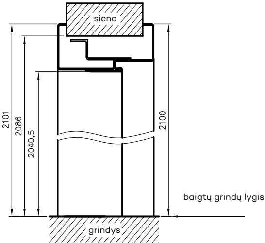
Vertikalus pjūvis OSRB
