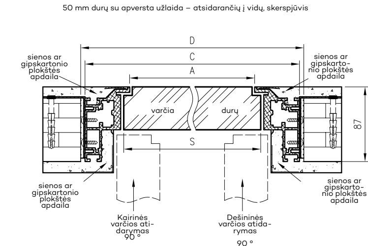
„Profi“ durų pločio matmenys
