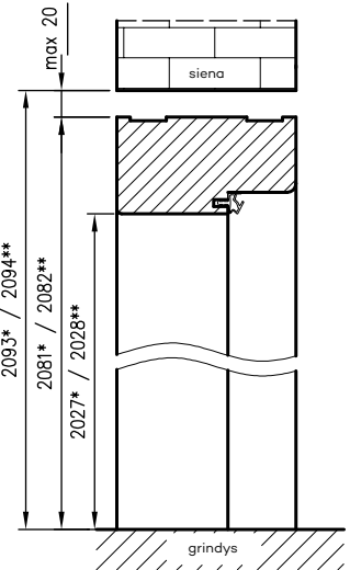
Stiklinių durų su ORC vertikalus pjūvis priešgaisrinės durys
