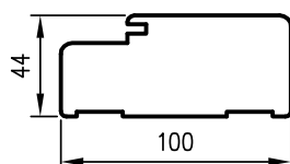
OP profilis
