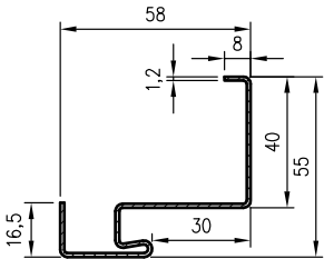
OSMK staktos profilis
