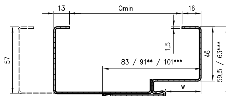
OSR staktos profilis su T57 uždarymo kampiniu
