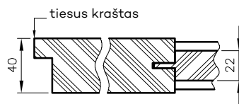
Horizontalus Elsa durų pjūvis
