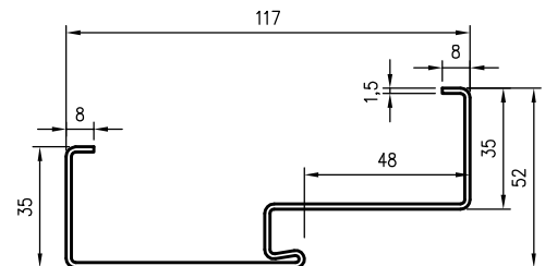
Staktos profilis
