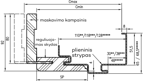
Staktos profilis
