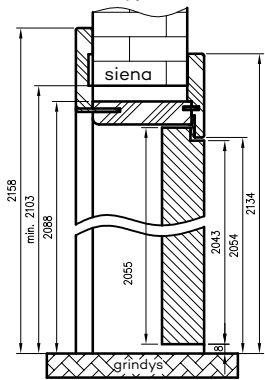
Vertikalus pjūvis ORO
