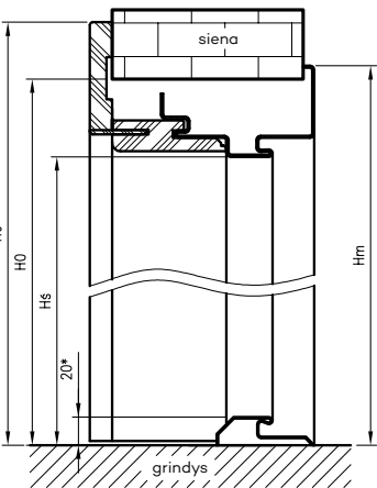
OSH STAND matmenys dvivėrėms durims
