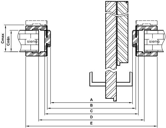
Sulankstomų durų atidarytoje padėtyje skerspjūvis
