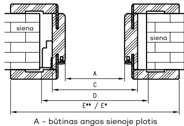
Horizontalus pjūvis OR/ORC
