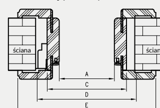
Przekrój poziomy OR/ORC
