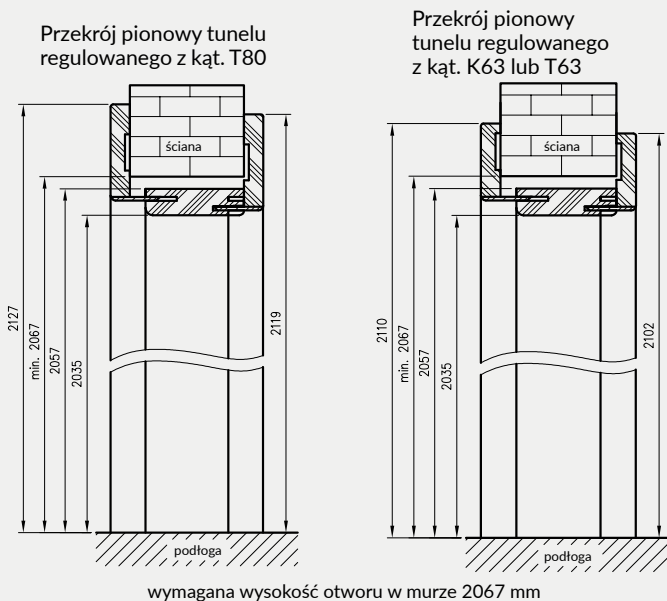
Przekrój poprzeczny TUN
