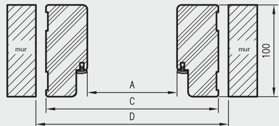
Przekrój poziomy OP
