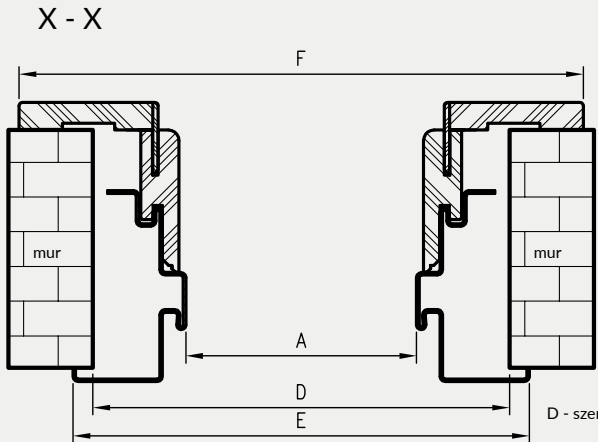
Profil ościeżnicy
