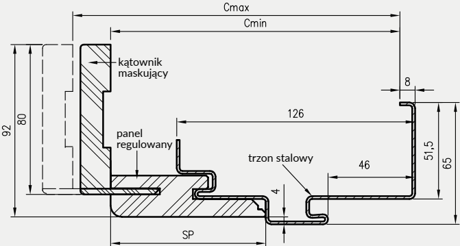
Profil ościeżnicy OSHB
