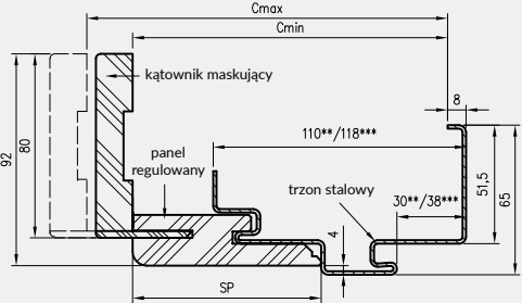
Profil ościeżnicy
