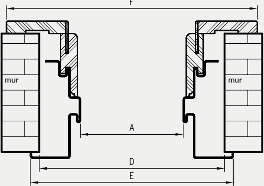
Przekrój poziomy OSHB
