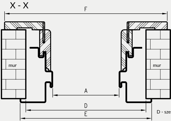
Profil ościeżnicy
