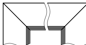
varianta zárubně spojované pod úhlem: 90°
