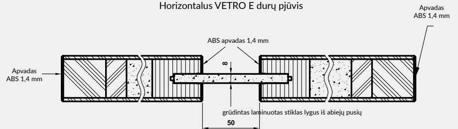
Horizontalus VETRO E durų pjūvis
