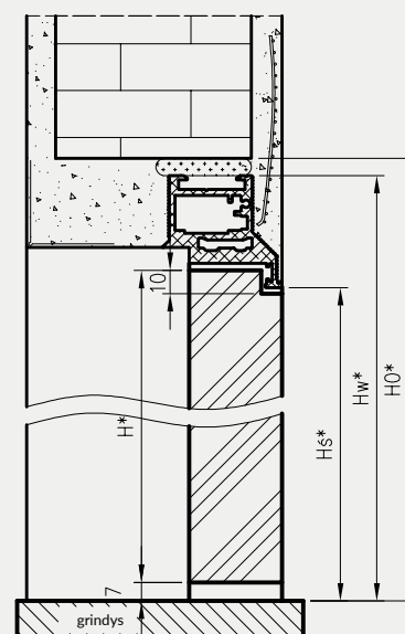
Sara Eco 2 durų su apversta užlaida – atsidarančių į vidų, vertikalus pjūvis
