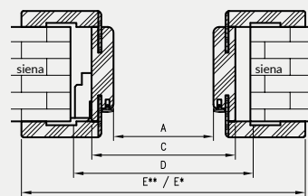
Horizontalus pjūvis OR/ORC
