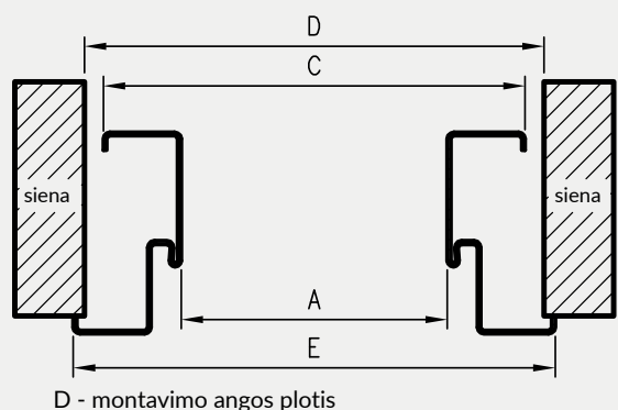
D - montavimo anġs plotis
