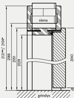
Stiklinių durų su ORC vertikalus pjūvis stiklinės durys
