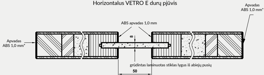
Horizontalus VETRO E durų pjūvis
