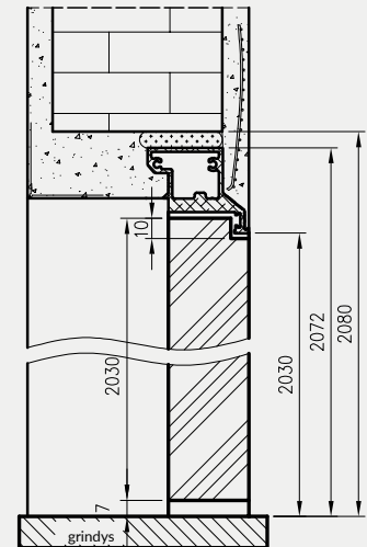
Sara Eco 2 durų su apversta užlaida – atsidarančių į vidų, vertikalus pjūvis
