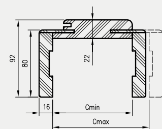
OR su kamp. T80 pjūvis
