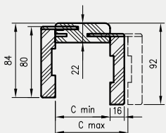
TUN su kamp. T63 pjūvis
