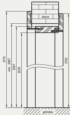
Reguliuojamo tunelio su kamp. T63 vertikalus pjūvis
