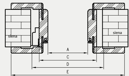
Horizontalus pjūvis OR
