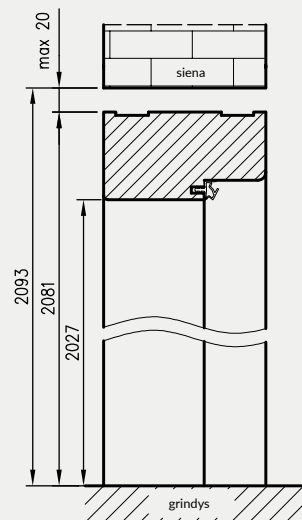
Vertikalus pjūvis priešgaisrinės durys
