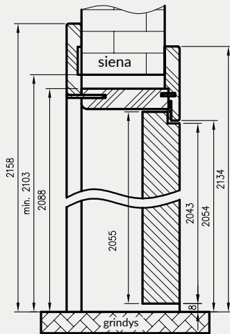
Vertikalūs pjūvis ORO
