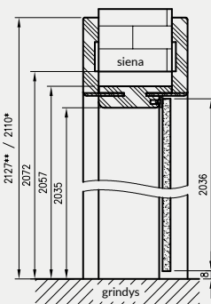
Stiklinių durų su ORC vertikalus pjūvis stiklinės durys
