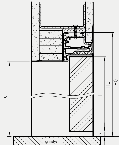
Sara Eco 2 lygiabriaunių durų – atsidarančių į išorę, vertikalus pjūvis
