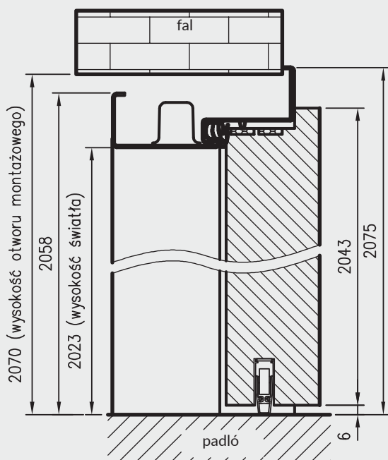
Olimp EI60 méretek egyszárnyú ajtókhöz
