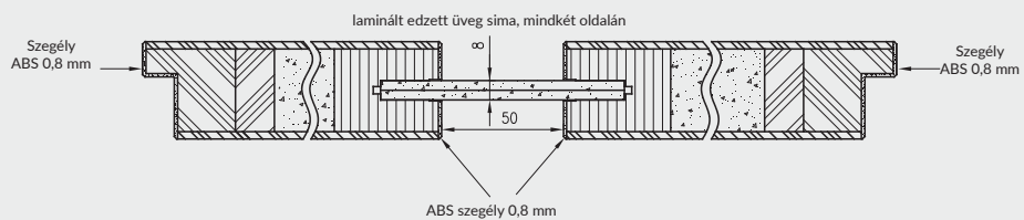
VETRO E falc nélküli ajtó vízszintes metszete
