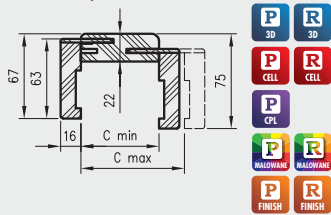
TUN záróprofilal metszete T63
