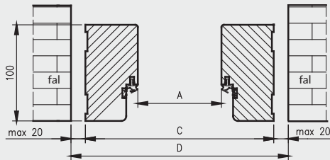
OD méretek Athos ajtóhoz
