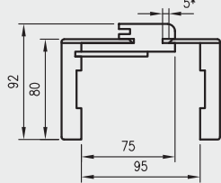
ORB 075 keresztmetszet
