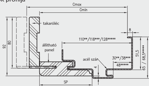
tok profilja
