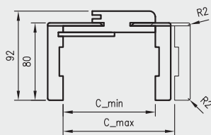
ORB 075 keresztmetszet 5*
