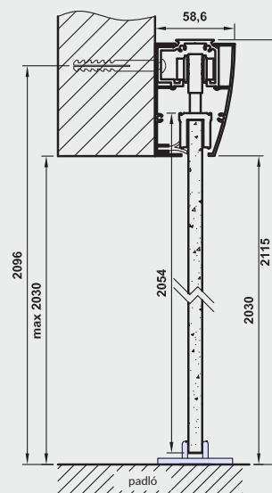
A - A függőleges Spazio TO rendszer keresztmetszet
