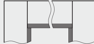
ORB 90°-os csatlakozás T80 záróprofil
