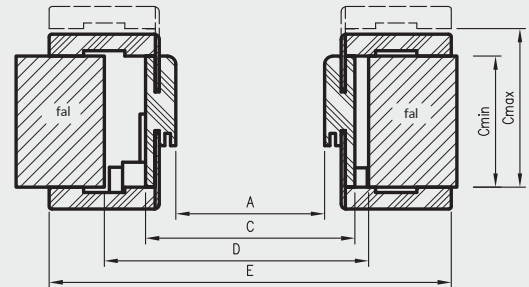
Vízszintes ORB keresztmetszet
