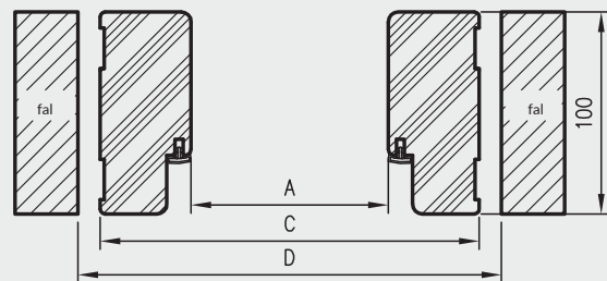
Vízszintes keresztmetszet OP
