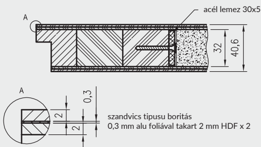
betörésgátló Solid RC2 ajtólap
