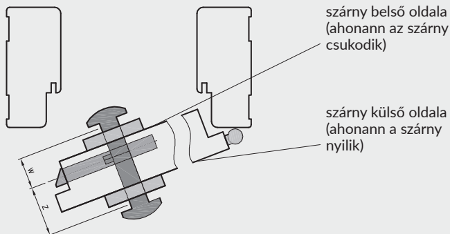
Rajz . gömbös zárbetét méretének kiválasztása
