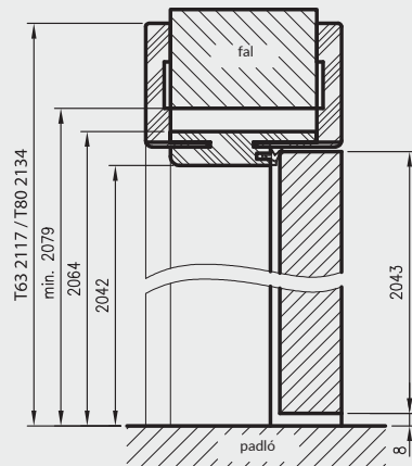
Optimális falnyílás magasság 2073mm
