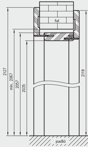
Az állítható átjárótok záróprofilal függőleges metszete T80
