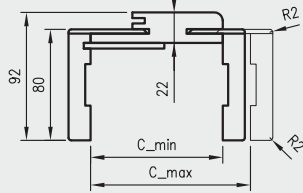
ORB 075 keresztmetszet
