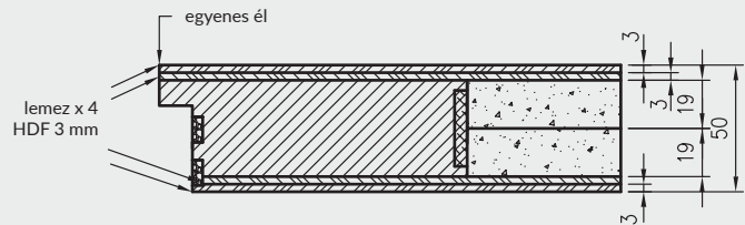
Tűzajtó szárny Athos EI30
