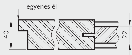
Viszszintes Elsa ajtópanel keresztmetszet
