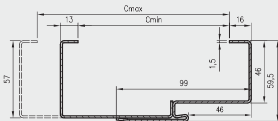
OSRB ajtótok profilja
