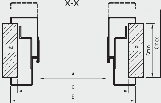
OSRB vízszintes metszet
