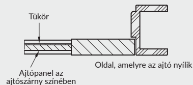
Estra 10 ajtó „Hátlap” változatban
