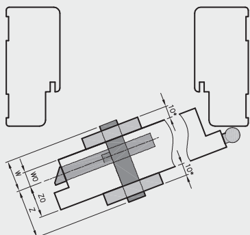
Rajz . zárbetét méretének kiválasztása
