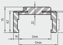
OR/ORC metszet záróprofil T63
