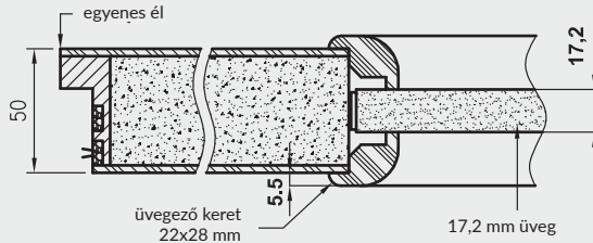
Tűzajtó szárny Olimp EI30
