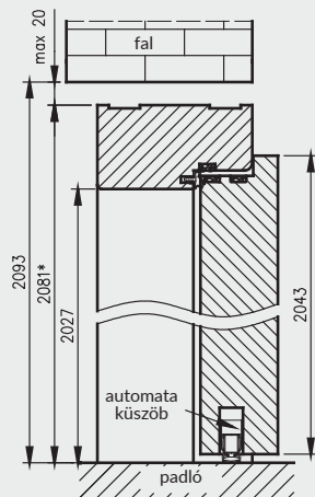
Athos ajtó fa ajtók Takaró tömítéssel*
