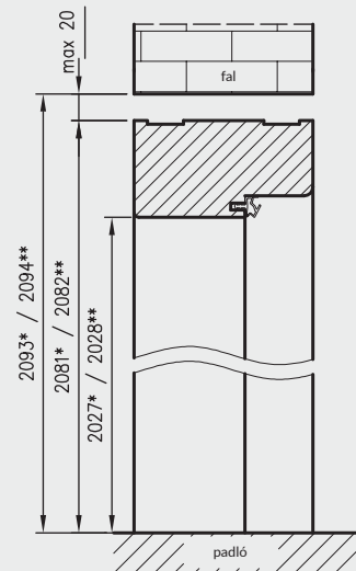
Függőleges keresztmetszet tűzgátló ajtó.
