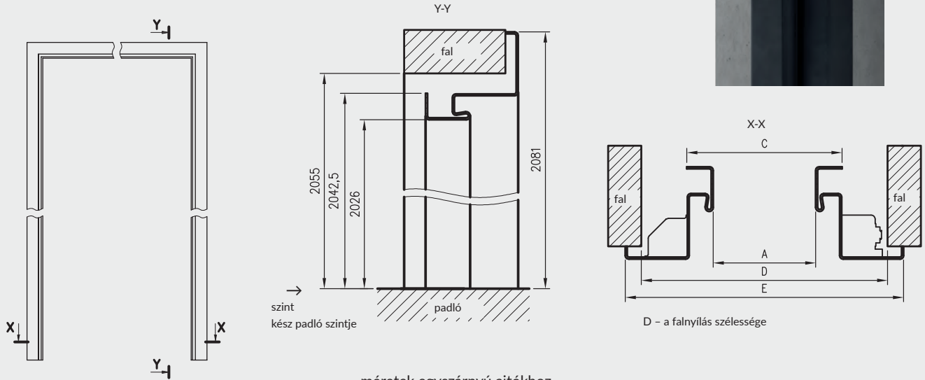
méretetek egyszárnyú ajtókhöz
