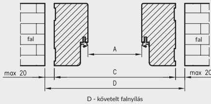
Viszszintes keresztmetszet falban szerelt tok
