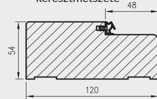
OLIMP EI60 ajtókhöz való fa ajtótok keresztmetszete
