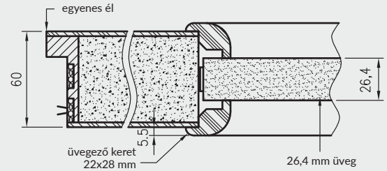
Tűzajtó szárny Olimp EI60
