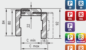
TUN záróprofilal metszete T63
