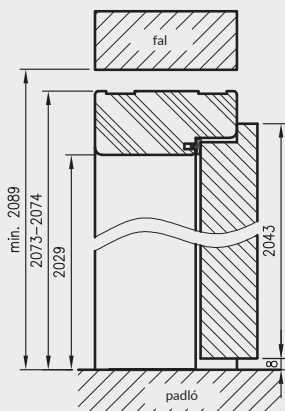
Függőleges keresztmetszet OP falcolt ajtók
