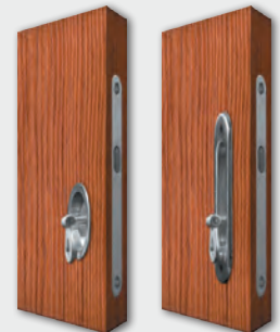
Horgos zár kulccsal és fogantyúval kerek
