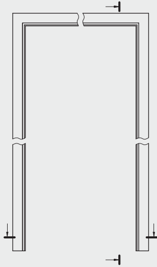
OSRB vízszintes metszet
