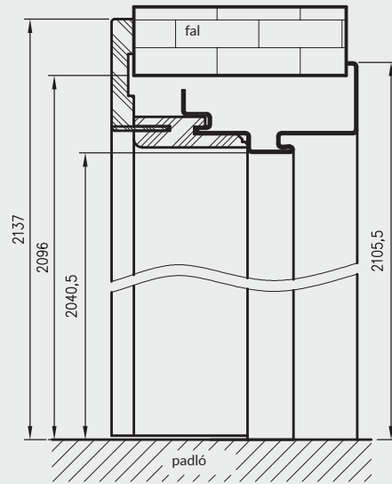
Y-Y OSHB függőleges metszet
