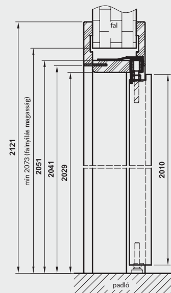
Függőleges keresztmetszet
