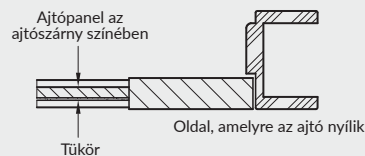
Estra 10 ajtó „Hátlap” változatban
