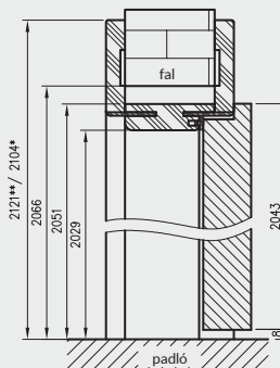
Függőleges keresztmetszet üvegajtók ORC
