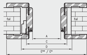
D - szükséges falnyílás szélesség
