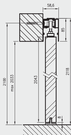
Függőleges keresztmetszet
