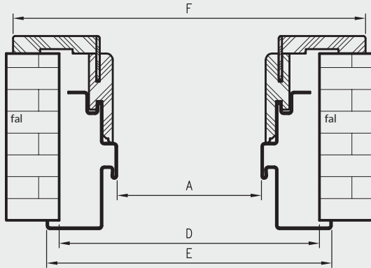
OSHB vízszintes metszet X-X
