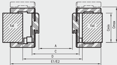
Vízszintes ORB keresztmetszet
