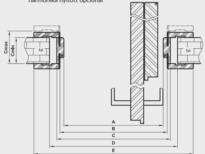
ajtó átlós keresztmetszete harmonika nyitott opciónál *
