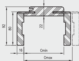
OR/ORC metszet záróprofil T80
