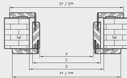
átlós TUN keresztmetszet
