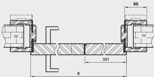
Átlós keresztmetszet zárt opciónál (jobb ajtó, bal ajtó tükrös képe)
