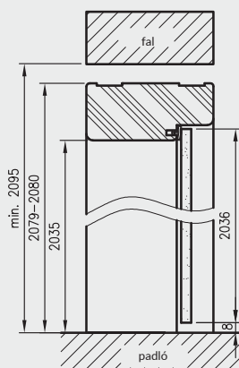
Függőleges keresztmetszet OP Üveg ajtók
