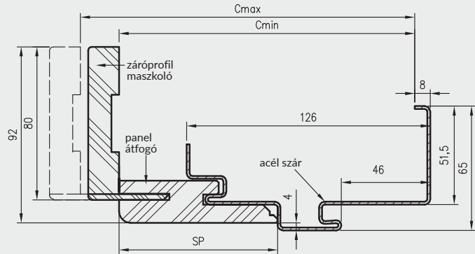
OSHB ajtótok profil
