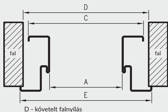
OSS szélességi méretek
