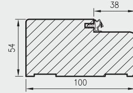
OLIMP EI60 ajtókhöz való fa ajtótok keresztmetszete
