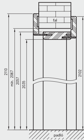
Az állítható átjárótok záróprofilal függőleges metszete T63
