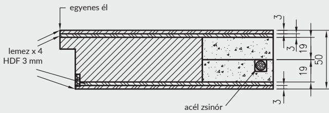
Lopásgátló ajtó és tűzvédelmi ajtó Forca EI30
