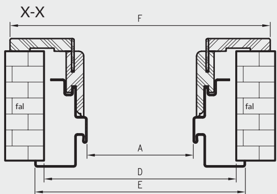
tok profilja
