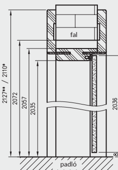
Függőleges keresztmetszet üvegajtók ORC
