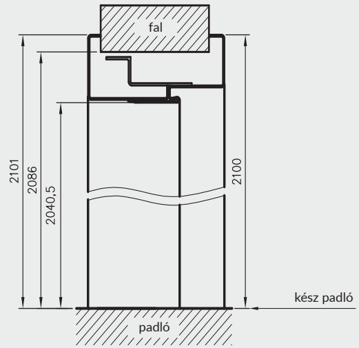
OSRB függőleges metszet
