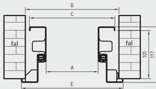
D - követelt falnyílás
