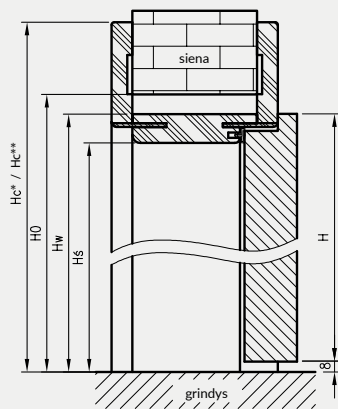
Vertikalus pjūvis OR
