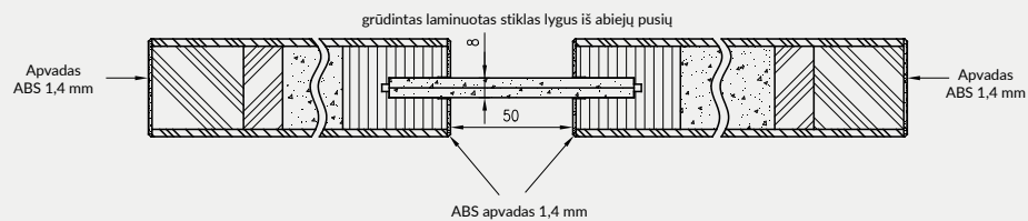
Horizontalus VETRO E durų pjūvis
