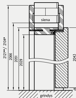
Stiklinių durų su ORC vertikalus pjūvis stiklinės durys iš ORC
