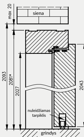
Medinė stakta „Athos“ durims su nuleidžiamu tarpikliu*
