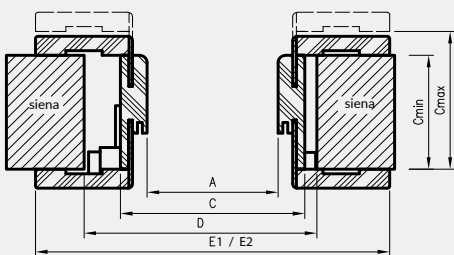
Horizontalus pjūvis ORB
