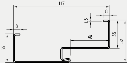
Staktos profilis
