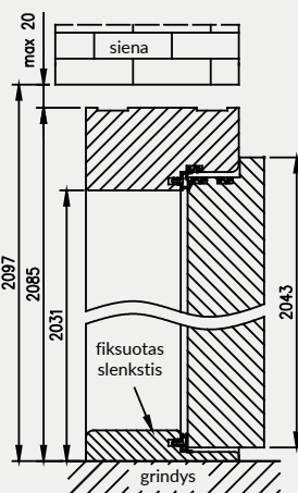
Medinė stakta „Athos“ durims su fiksuotu slenksčiu
