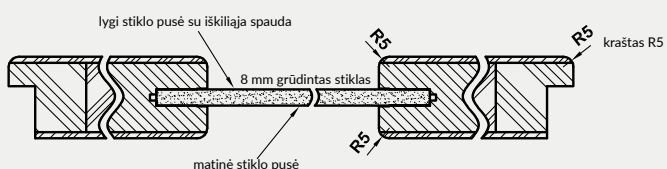
Horizontalus VETRO B5, B10-B11 durų pjūvis
