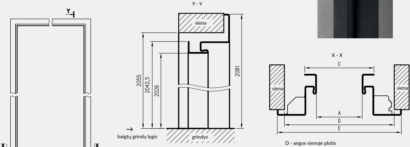
matmenys vienvėrėms durims
