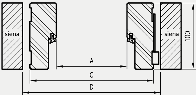
horizontalus pjūvis OPB
