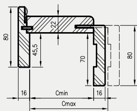
Staktos profilis
