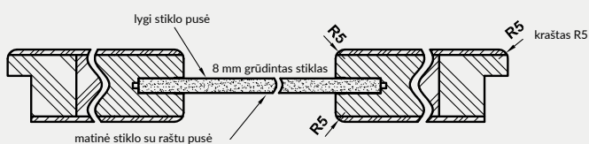
Horizontalus VETRO A5, A10-A11 durų pjūvis
