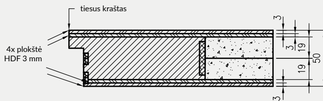
„Athos EI30“ priešgaisrinė durų varčia
