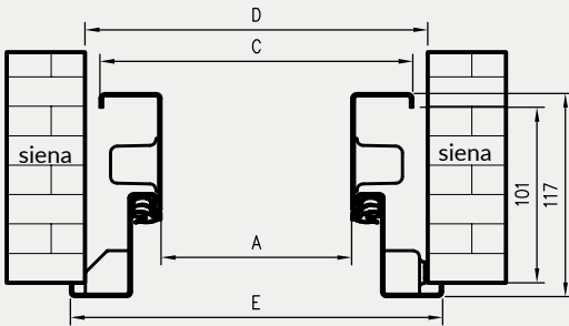
D - montavimo angos plotis
