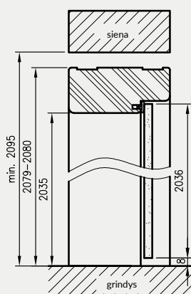
Vertikalus pjūvis OP stiklinėms durims
