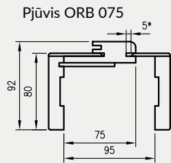
Horizontalus pjūvis ORB
