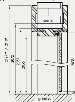
Stiklinių durų su ORC vertikalus pjūvis stiklinės durys iš ORC
