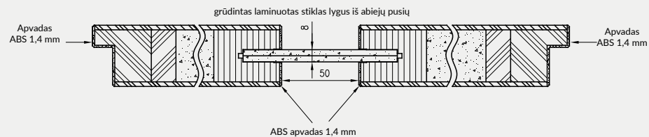
Horizontalus VETRO E durų pjūvis
