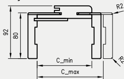
Pjūvis ORB 075
