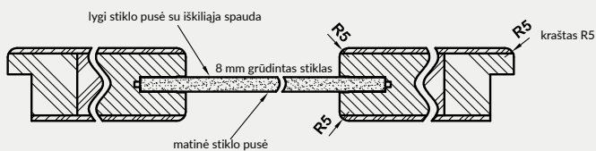
Horizontalus VETRO A5, A10-A11 durų pjūvis
