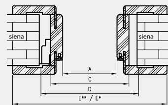
Horizontalus pjūvis OR/ORC
