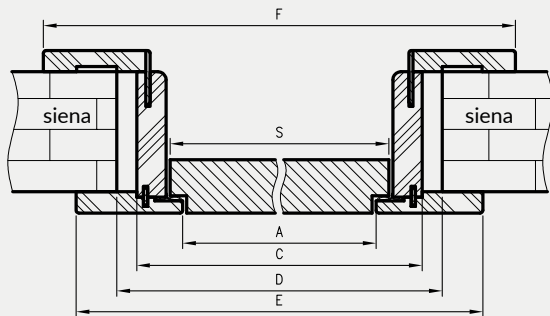
Horizontalus pjūvis ORO
