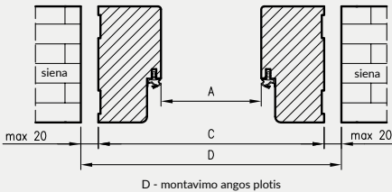
Durų staktos sienoje horizontalus pjūvis durų rėmas sienoje
