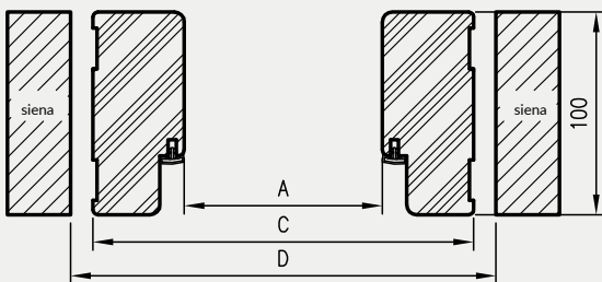
Horizontalus pjūvis OP
