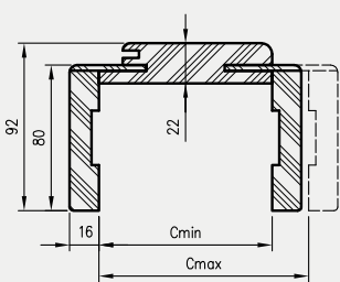
OR su kamp. T80 pjūvis
