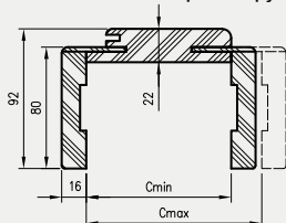
OR/ORC su kamp. T80 pjūvis
