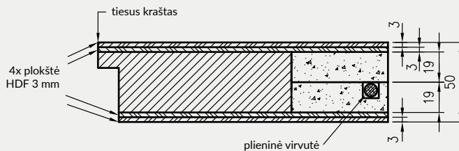
„Forca B“ priešsilaužiminė durų varčia
