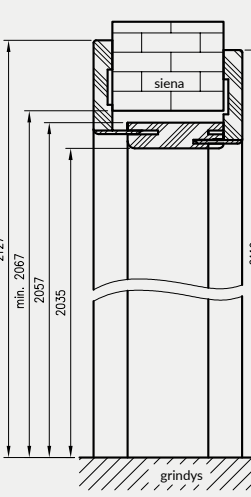
Reguliuojamo tunelio su kamp. T80 vertikalus pjūvis
