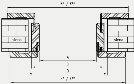
TUN skerspjūvis
