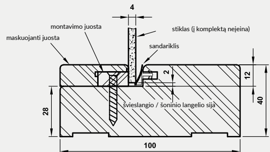
Švieslangių/šoninių langelių matmenų lentelė
