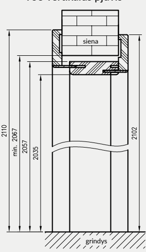
Reguliuojamo tunelio su kamp. T63 vertikalus pjūvis
