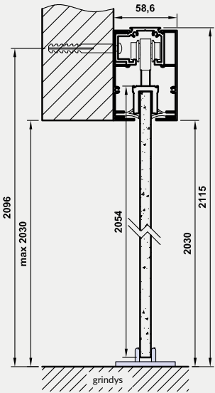
A – vertikalus „Spazio TP“ sistemos vertikalus pjūvis
