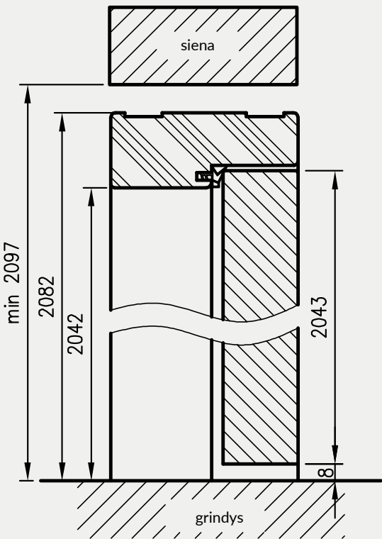
Vertikalus pjūvis OPB
