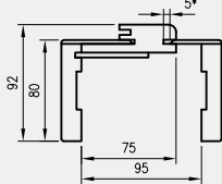
Pjūvis ORB 075
