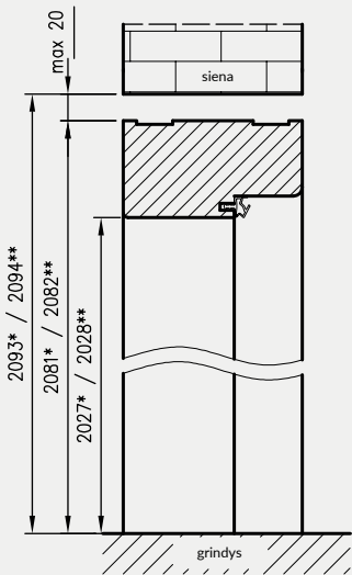
Užlaidinių durų su OR vertikalus pjūvis priešgaisrinės durys
