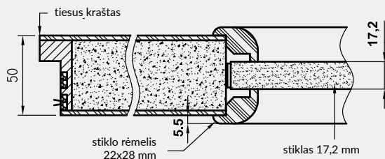
Olimp EI30 ugniai priešgaisrinė durų varčia
