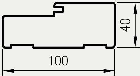
OPB profilis
