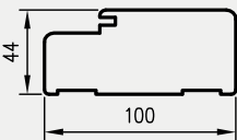
profilis OP SOFT
