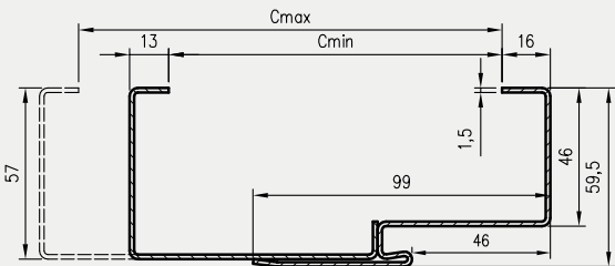
OSRB staktos profilis
