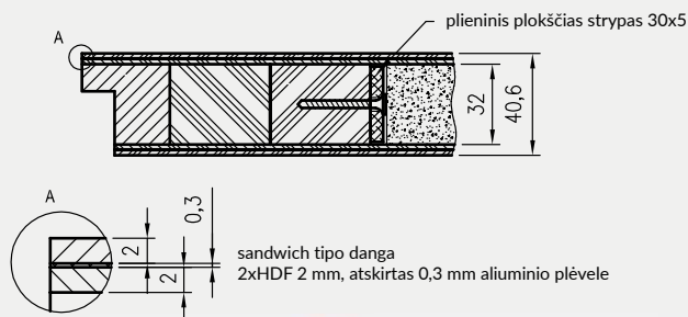
„Solid RC2“ priešsilaužiminė durų varčia
