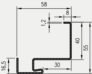
OSMK staktos profilis
