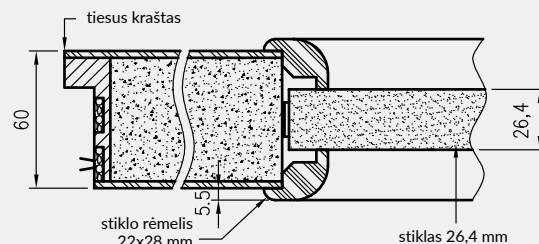
Olimp EI60 ugniai priešgaisrinė durų varčia
