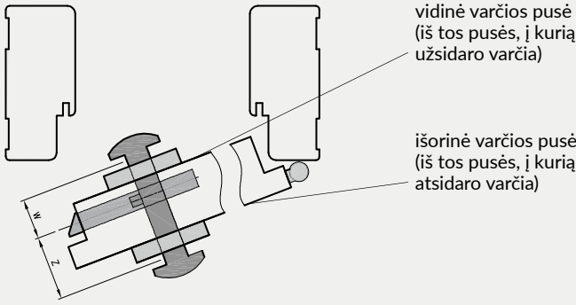
Pav. Cilindro su rankena dydžio pasirinkimas
