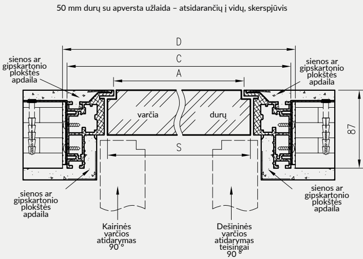
„Profi“ durų pločio matmenys
