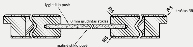
Horizontalus VETRO D1 durų pjūvis
