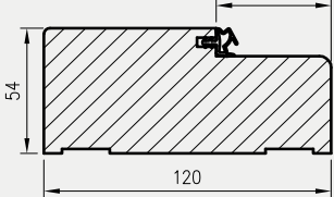
OLIMP EI60 durų medinio staktos pjūvis
