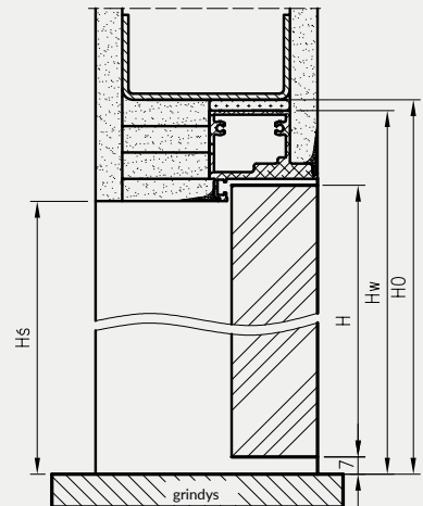
DRE profilis į išorę atsidarančioms lygiabriaunėms durims
