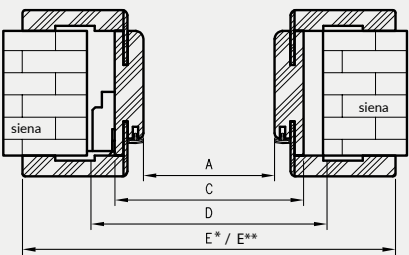
Horizontalus pjūvis OR
