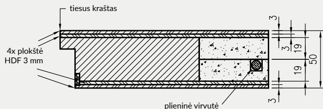
„Forca EI30“ priešsilaužiminė priešgaisrinė durų varčia
