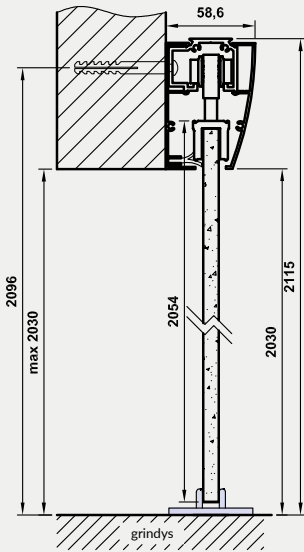
A – vertikalus „Spazio TO“ sistemos vertikalus pjūvis
