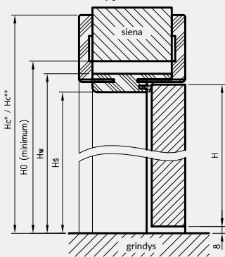
Vertikalus pjūvis ORB
