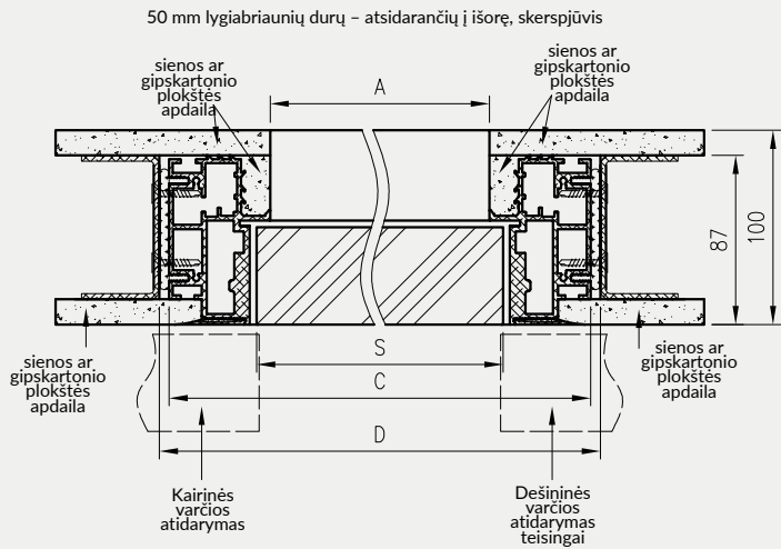
„Profi“ durų pločio matmenys
