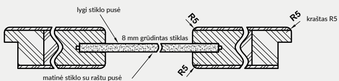
Horizontalus VETRO B5, B10-B11 durų pjūvis
