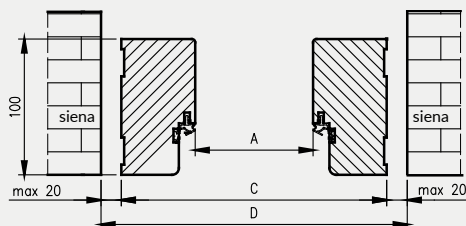
Athos durų OD matmenys
