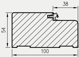
OLIMP EI60 durų medinio staktos pjūvis
