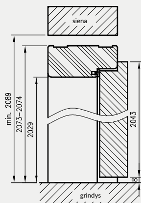
Vertikalus pjūvis OP užlaidinėms durims
