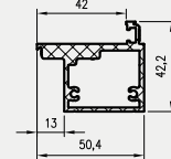
DRE profilis į išorę atsidarančioms lygiabriaunėms durims
