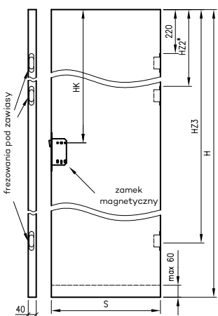
Skrzydła bezprzylgowe rozierne Standard 10, Modern, Plus
