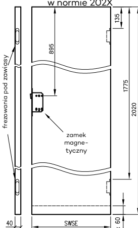
Skrzydła Sara Eco 2 bezprzylgowe w normie 202X
