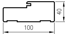
OPB profile
