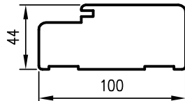
OP (fixed door frame) profile
