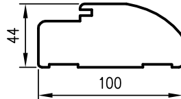
OP SOFT (fixed door frame SOFT) profile
