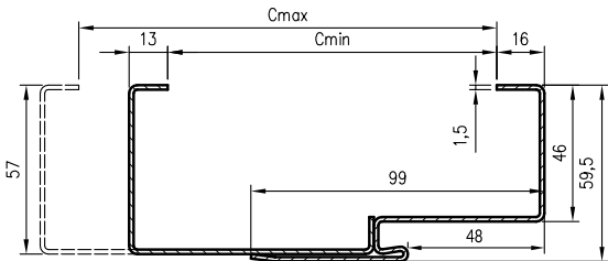
OSRB door frame profile
