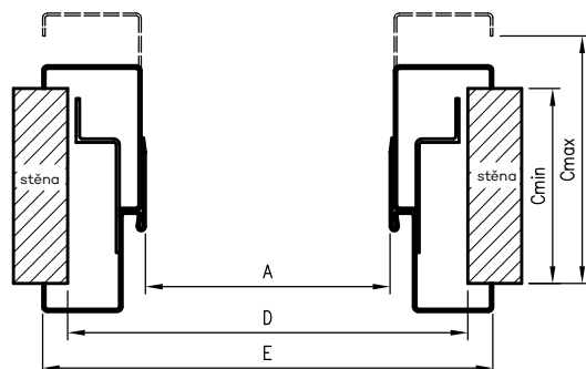
Vodorovný průřez OSRB
