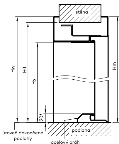
Profil rámu OSR s zavíracím úhelníkem T57
