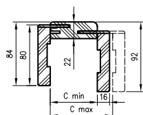
Průřez TUNEL s úhelníkem T63
