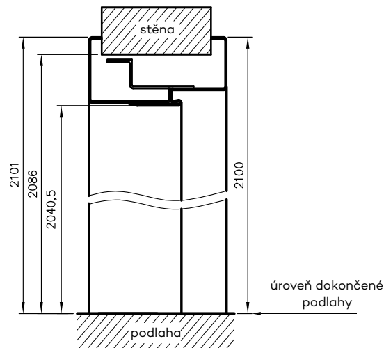
Svislý průřez OSRB
