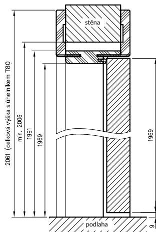
Svislý průřez ORB
