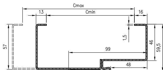
Profil zárubně OSRB
