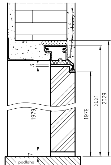
Profil DRE pro dveře s obráceným falcem otevírané dovnitř
