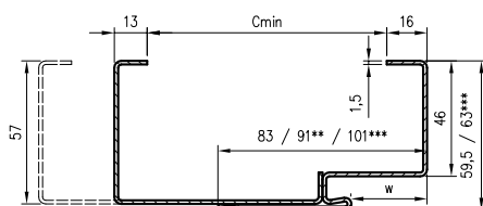
Profil rámu OSR s zavíracím úhelníkem T57
