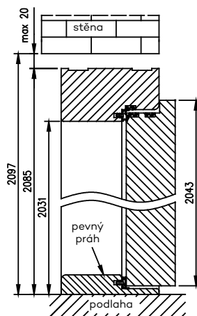
Dřevěná zárubeň dveří Athos s pevným prahem
