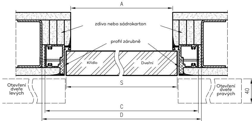
Příčný průřez pro bezfalcové dveře Sara Eco2 - otevírání směrem ven
