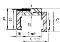
Průřez TUNEL s úhelníkem T63
