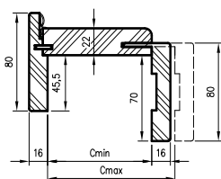
Profil zárubně
