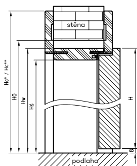
Svislý průřez OR
