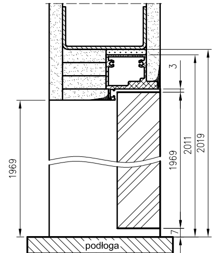
Svislý průřez pro dveře Sara Eco 2 bezfalcové - otevírání směrem ven
