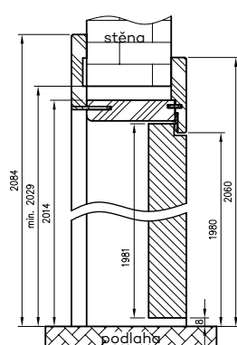
Svislý průřez ORO
