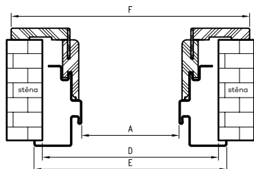
Profil zárubně
