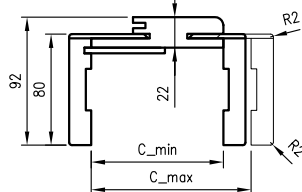
Průřez ORB 075
