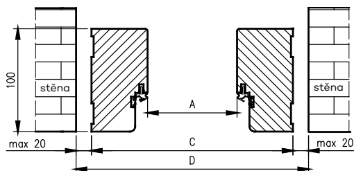
Rozměry OD pro dveře Athos
