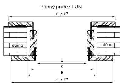
Průřez TUNEL s úhelníkem T80
