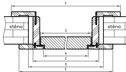
Horizontální řez ORO
