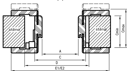
Vodorovný průřez ORB
