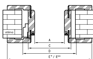
Vodorovný průřez OR
