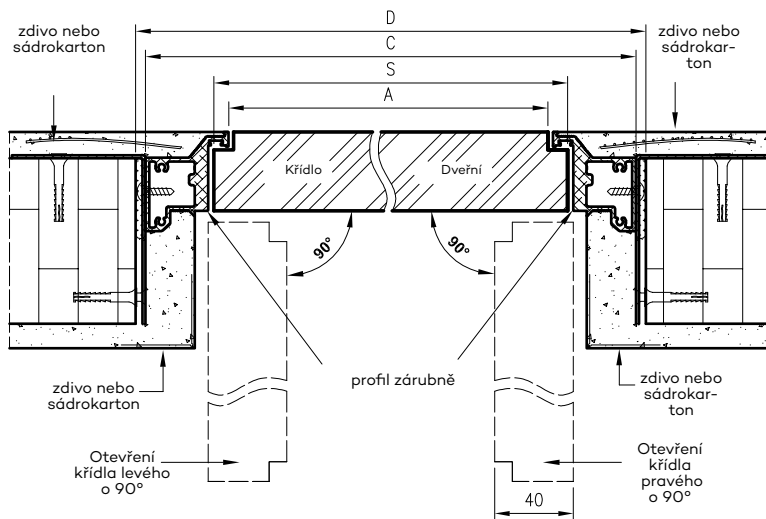
Příčný průřez dveří Sara Eco 2 s obráceným falcem - otevírání dovnitř
