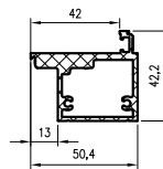
Profil DRE pro dveře otevírané v jedné rovině směrem ven
