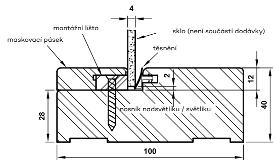
Tabulka rozměrů pro nadsvětlíky / boční světlíky
