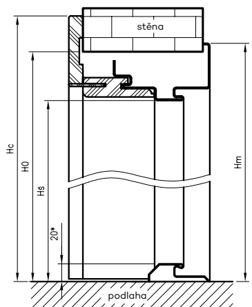
Rozměry OSH STAND pro dvoukřídlé dveře
