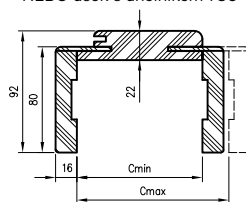
NEBO úsek s úhelníkem T80
