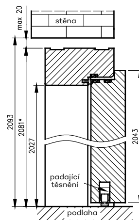
Dřevěná zárubeň dveří Athos s padajícím těsněním
