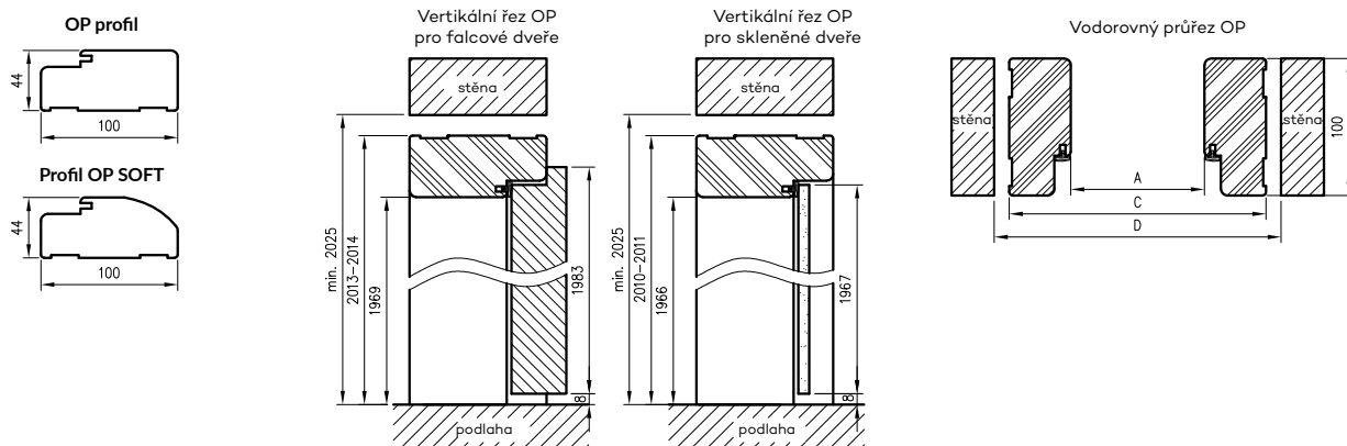
rovná zárubeň soft
