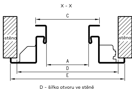
rozměry pro jednokřídlé dveře
