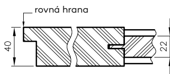
Vodorovný průřez dveří Elisa
