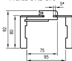
Průřez ORB 075
