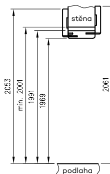
Příčný průřez TUNEL s úhelníkem T80
