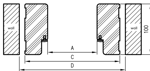
OP Horizontal cross section
