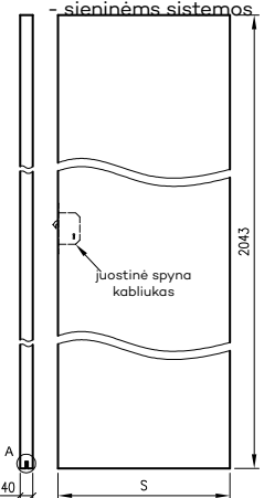
Stumdomos varčios skirtos: - PA staktinėms kasetėms - SPAZIO CD sistemoms - sieninėms sistemoms
