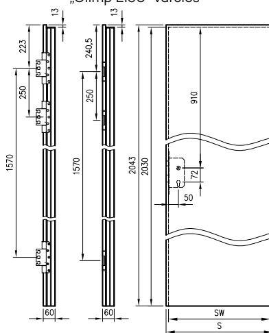
„Olimp EI60“ varčios**
