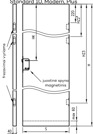
Atveriamos lygiabriaunės varčios Standard 10, Modern, Plus
