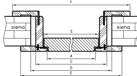
Horizontalus pjūvis ORO
