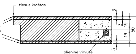
„Forca B“ priešsilaužiminė durų varčia
