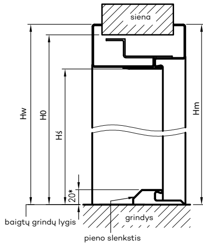
OSR staktos profilis su T57 uždarymo kampainiu
