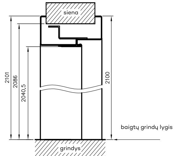
Vertikalus pjūvis OSRB
