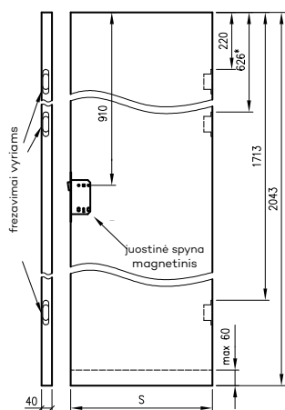
Atveriamos lygiabriaunės varčios
