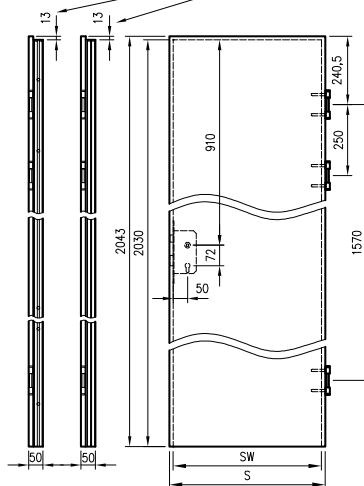
„Athos“ / „Olimp EI30“ varčios
