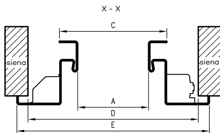
matmenys vienvėrėms durims
