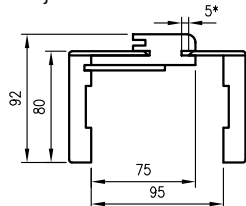
Pjūvis ORB 075
