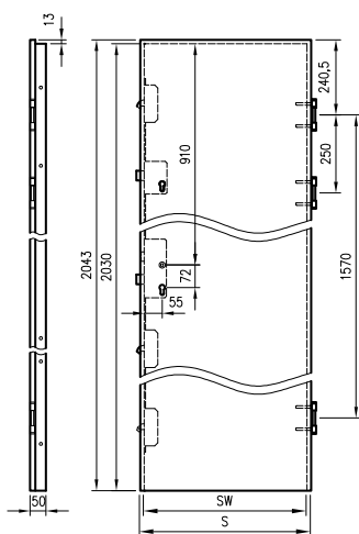
„Forca“ / „Forca B“ varčios
