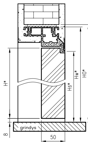
50 mm durų su apversta užlaida – atsidarančių į vidų, vertikalus pjūvis
