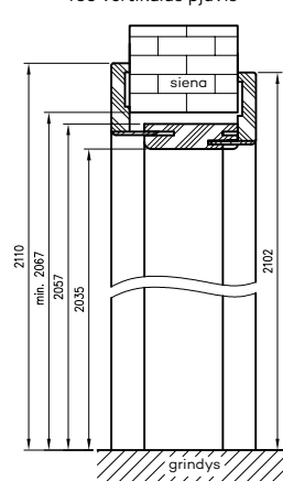
Reguliuojamo tunelio su kamp. T63 vertikalus pjūvis
