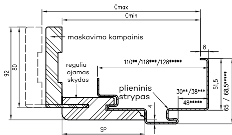
Staktos profilis
