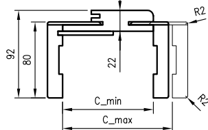
Pjūvis ORB 075
