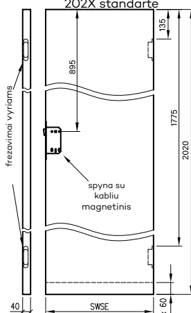
Varčios „Sara Eco“ 2 lygiabriaunės 202X standarte
