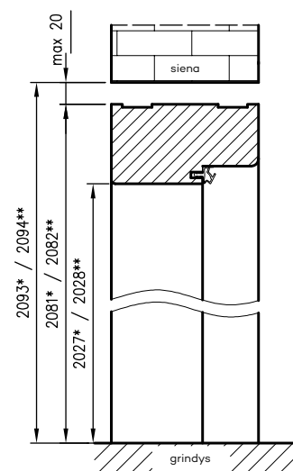
Stiklinių durų su ORC vertikalus pjūvis priešgaisirinės durys
