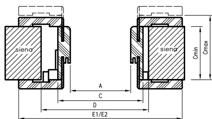
Horizontalus pjūvis ORB
