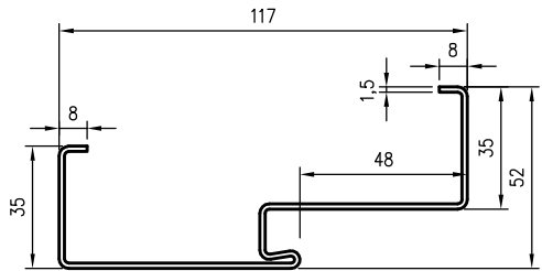
Profil ościeżnicy
