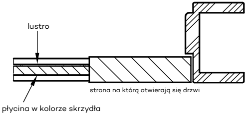
Drzwi ESTRA 10 bezprzylgowe lub przylgowe w wariantach "Rewers"
