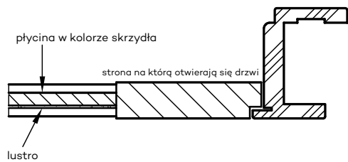
Drzwi ESTRA 10 z odwróconą przyłgą w wariantach "Rewers"
