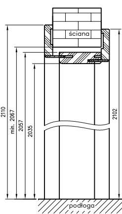
Przekrój pionowy tunelu regulowanego z kąt. T63
