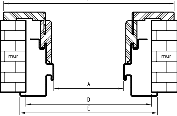
Profil ościeżnicy
