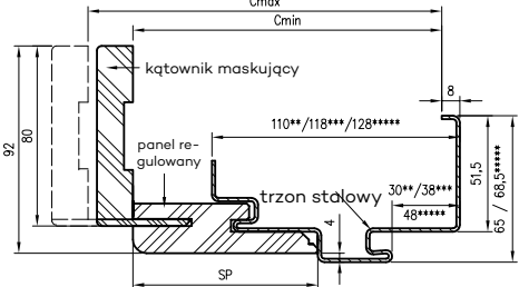
Profil ościeżnicy
