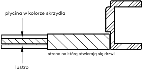
Drzwi ESTRA 10 bezprzylgowe lub przylgowe w wariantach "Rewers"
