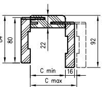
Przekrój TUN z kąt. T63
