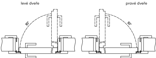
Profil zárubně
