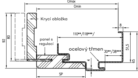
Profil zárubně
