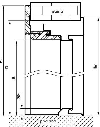
Rozměry HOZ STAND pro dvoukřídlové dveře
