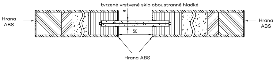
Vodorovný řez bezfalcovými dveřmi VETRO E
