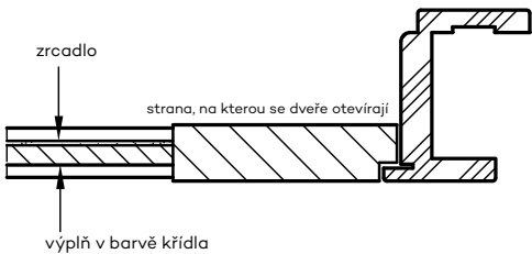
Dveře ESTRA 10 reverzní ve variantě „Reverz“
