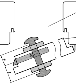
Obr. Výběr rozměru vložky s knoflíkem
