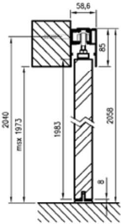
svislý řez
