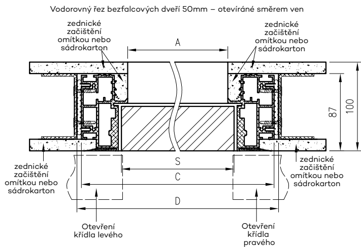
Rozměry šířky dveří Profi
