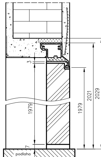
Profil DRE pro dveře reverzní otevírané dovnitř
