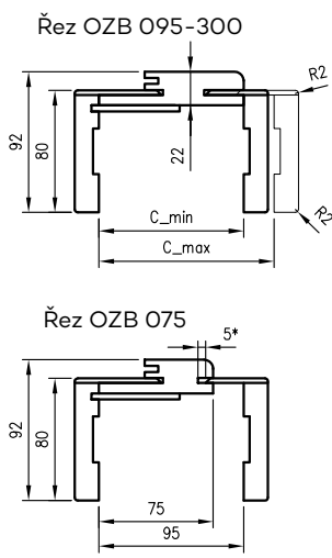
Vodorovný řez OZB
