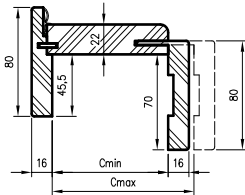
Profil zárubně
