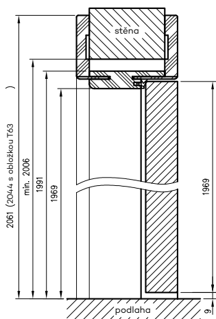
požadovaná výška stavebního otvoru 2006mm
