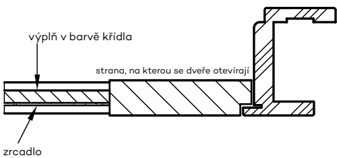
Dveře ESTRA 10 reverzní ve variantě „Reverz“
