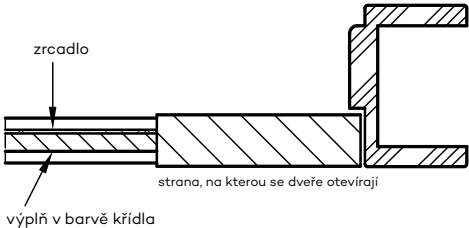
Dveře ESTRA 10 bezfalcové nebo falcové ve variantě „Reverz“
