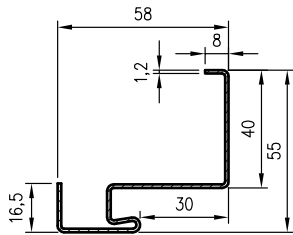
Profil zárubně OZMR
