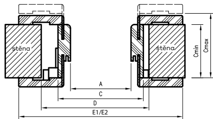
Vodorovný řez OZB
