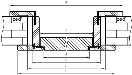
Vodorovný řez OZR
