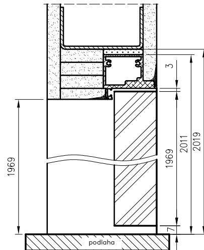
Svislý řez dveří Sara Eco 2 bezfalcové - otevírané směrem ven
