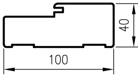
OPB profile
