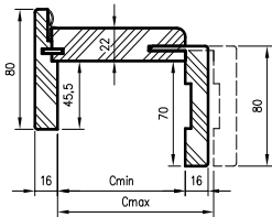
door frame profile
