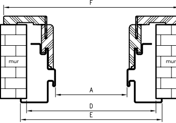
Profil ościeżnicy
