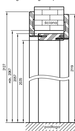
Przekrój pionowy tunelu regulowanego z kąt. T80
