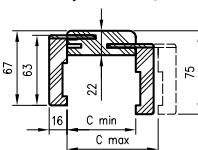
Przekrój TUN z kąt. T63
