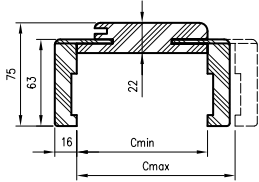
OR/ORC su kamp. T63 pjūvis
