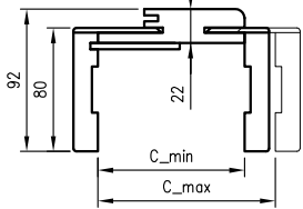
Pjūvis ORB 075
