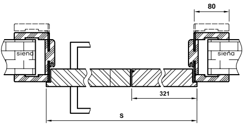
Sulankstomų durų uždarytoje padėtyje skerspjūvis (dešinės durys, kairinės durys yra veidrodinis vaizdas)
