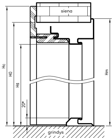
OSH STAND matmenys dvivėrėms durims
