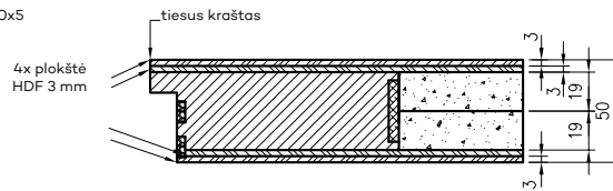
„Athos EI30“ priešgaisrinė durų varčia
