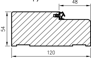
OLIMP EI60 durų medinio staktos pjūvis
