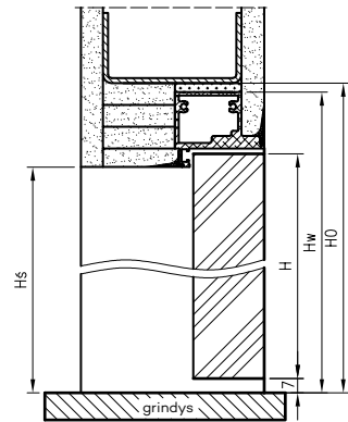
DRE profilis ī īšorē atsidarančioms lygiabriauņēms durims
