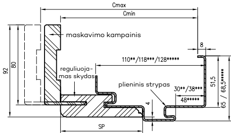
Staktos profilis
