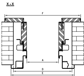
D - montavimo angos plotis
