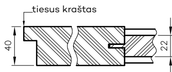
Horizontalus Elsa durų pjūvis
