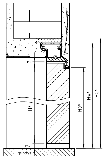
DRE profilis j vidų atsidarančioms durims su apversta užlaida
