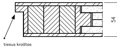
NEFRYT RC3 apsaugos nuo įsilaužimo durų varčia
