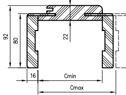
OR/ORC su kamp. T80 pjūvis
