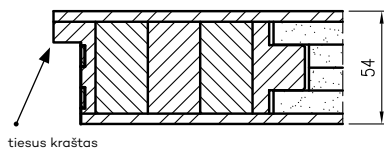
NEFRYT RC3 EI-30 apsaugos nuo įsilaužimo ir ugnies durų varčia
