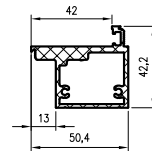
DRE profilis ī īšorē atsidarančioms lygiabriauņēms durims
