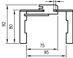
Horizontalus pjūvis ORB
