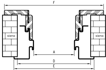
Staktos profilis
