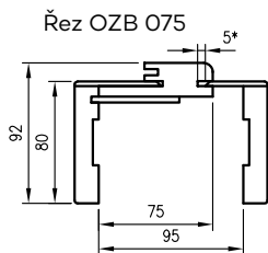
Vodorovný řez OZB
