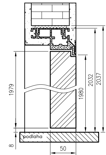
Svislý řez reverzních dveří 50 mm – otevírané směrem dovnitř
