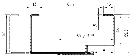
Profil rámu OZsR s krycí obložkou T57
