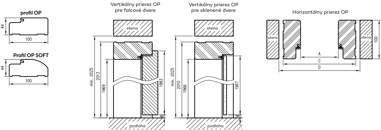
rovna zárubňa soft
