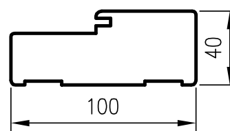
Profil OPB
