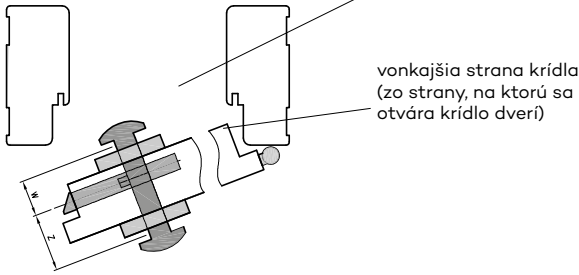
Obr. Výber veľkosti vložky s gombíkom
