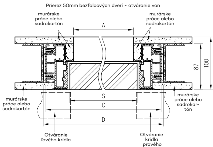
Rozmery šírky dvere Profi
