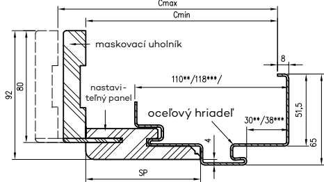
Profil zárubne
