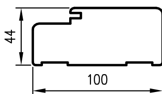
Profil OP
