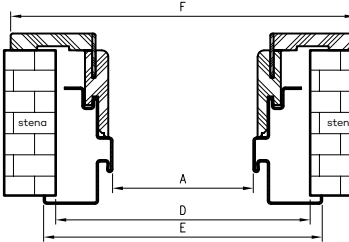
Profil zárubne
