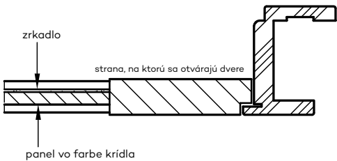
Dvere ESTRA 10 s reverzným falcom vo variante „Reverz“.
