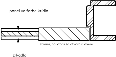
Dvere ESTRA 10 bezfalcové alebo falcové vo variante „Reverz“.
