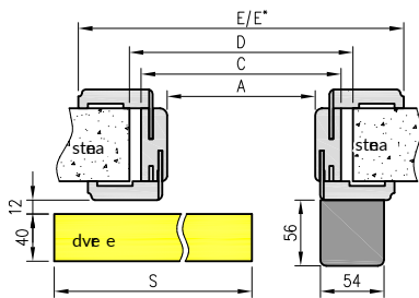
NT - horizontálny prierez (ľavý systém)
