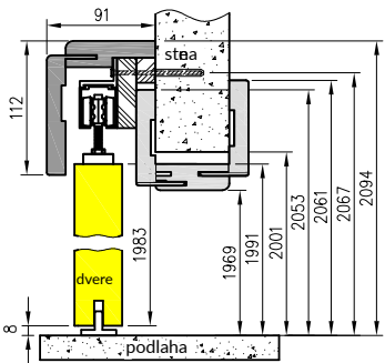
NT - vertikálny prierez na tuneli s uhl. 80 mm
