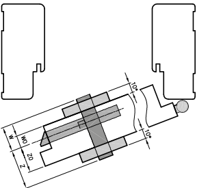
Obr. Výber veľkosti vložky valca
