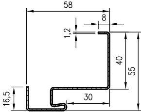
Profil zárubne OSMK
