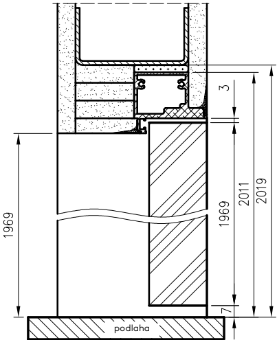
Vertikálna sekcia pre dvere Sara Eco 2 befalcové - otvárané smerom von
