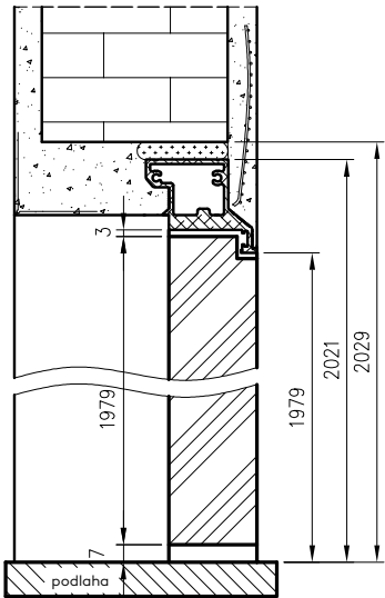
DRE profil pre dovnútra otvá- ateľné reverzné falcové dvere
