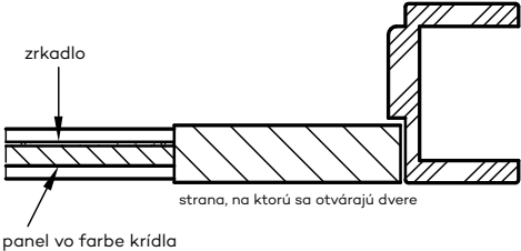
Dvere ESTRA 10 bezfalcové alebo falcové vo variante „Reverz“.
