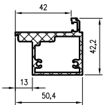
Profil DRE pre bezfalcové dvere otvárané von
