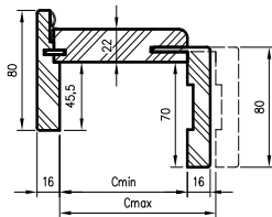
Profil zárubne
