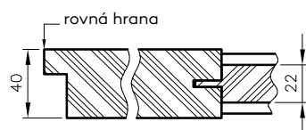
Horizontálny prierez dverí Elsa
