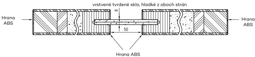
Vodorovný prierez bezfalcových dverí VETRO E
