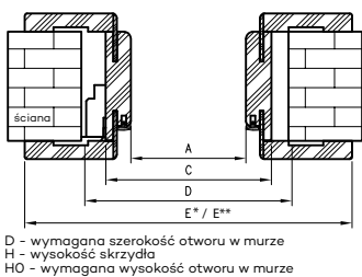
Przekrój OR z ką. T80
