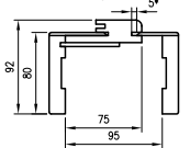
Przekrój ORB 075
