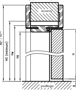
Przekrój pionowy ORB
