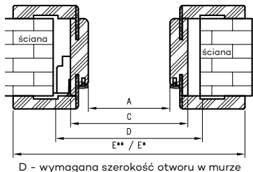
Przekrój poziomy OR/ORC
