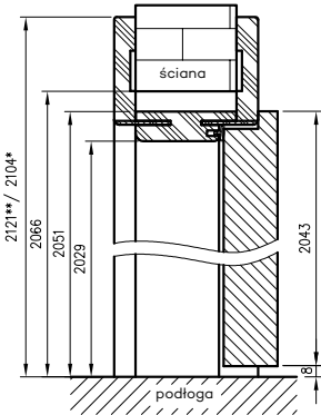
Przekrój pionowy drzwi przylgowych z OR
