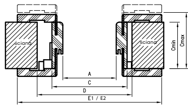
Przekrój poziomy ORB
