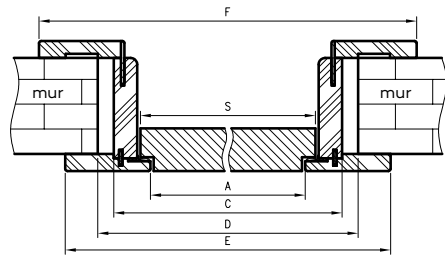
Przekrój poziomy ORO
